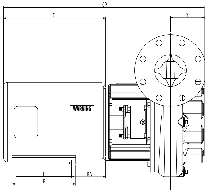
DIMENSIONS
