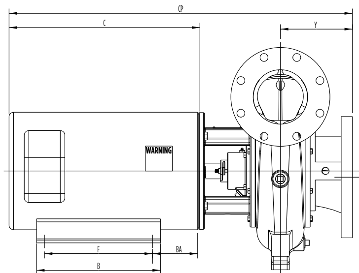
DIMENSIONS
